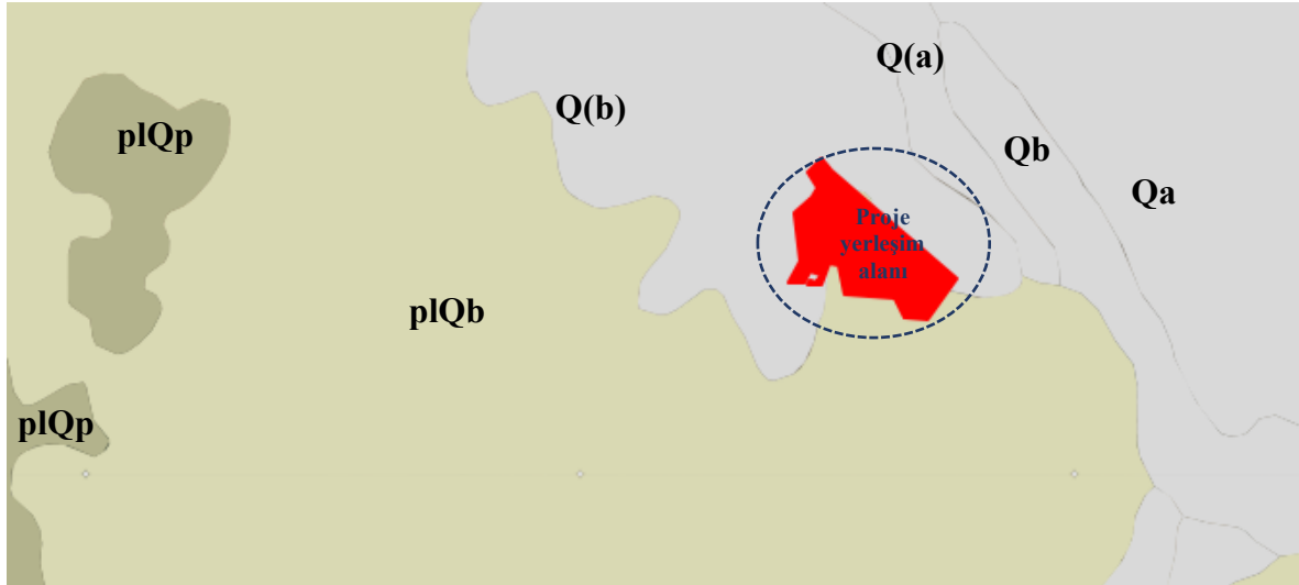
j1 - 2Şekil 5 .GES ve Yakın Çevresinin Genel Jeolojisi
